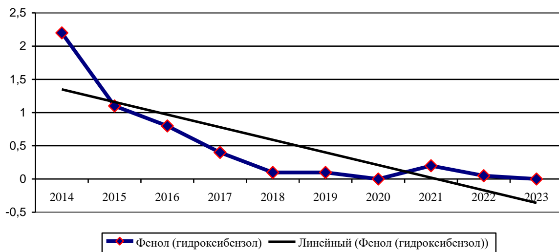
Рисунок 2 – Удельный вес проб воздуха фенола (гидроксибензола), превышающих предельно-допустимые концентрации в атмосферном воздухе г.Могилева в 2014–2023гг. по данным стационарных постов наблюдения филиала «Могилевоблгидромет»
