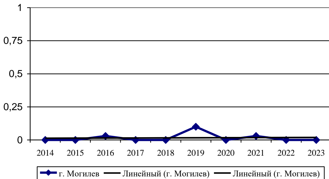
Рисунок 1 – Удельный вес проб воздуха углерода оксида (окись углерода, угарный газ), превышающих предельно-допустимые концентрации в атмосферном воздухе г.Могилева в 2014–2023гг по данным стационарных постов наблюдения филиала «Могилевоблгидромет»
